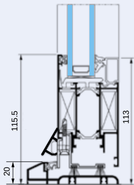
Seuil PMR démontable de 20 mm "bâtiment" pour une ouverture intérieure et extérieure
