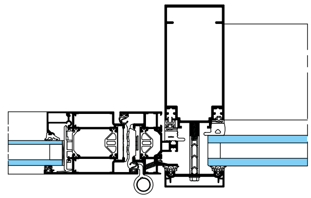
INTÉGRATION PORTE SOLEAL 65 SUR LA FAÇADE SPINAL
