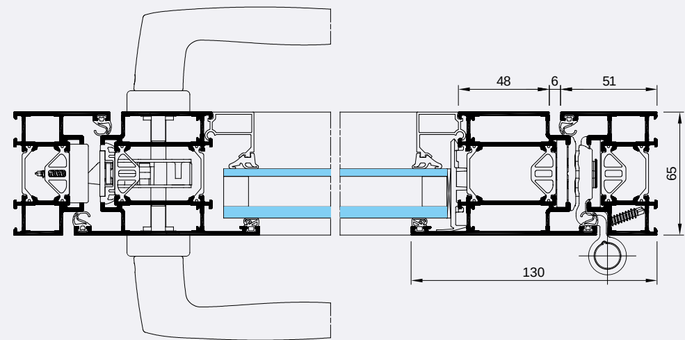
PORTE 1 VANTAIL OUVERTURE EXTÉRIURE
