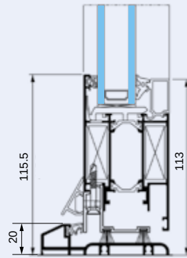
Seuil PMR de 20 mm "résidentiel", ouverture intérieure uniquement
