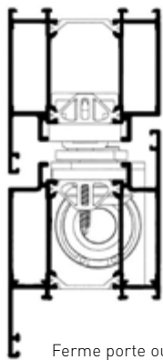
Ferme porte ouvrant
